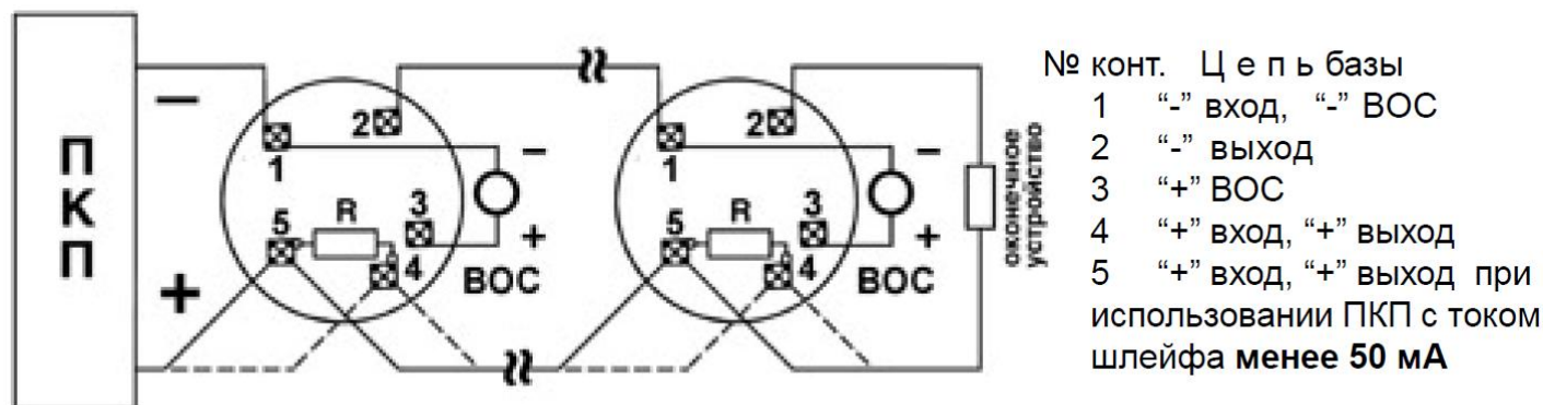
Рис.1. Схема подключения извещателей ИП101-23М-А1R с базами E1000R, E1000B к ПКП. Подключение с резистором показано пунктиром. В базе E1000B резистор и 4-й контакт не установлен.
